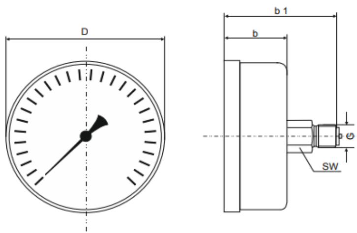
Baureihe 5641/5661
