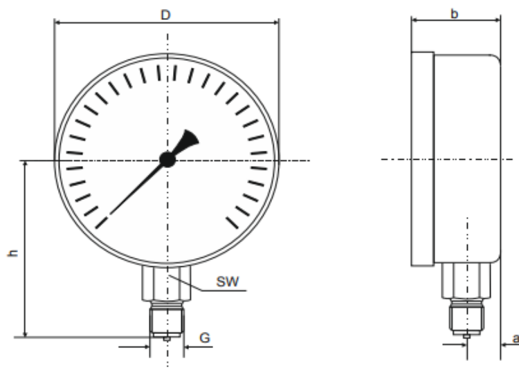
Baureihe 5631/5651
